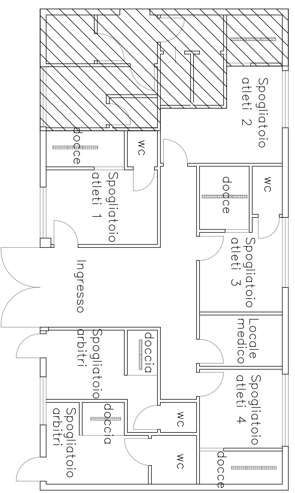
PLANIMETRIA SPOGLIATOI - scala 1:100
